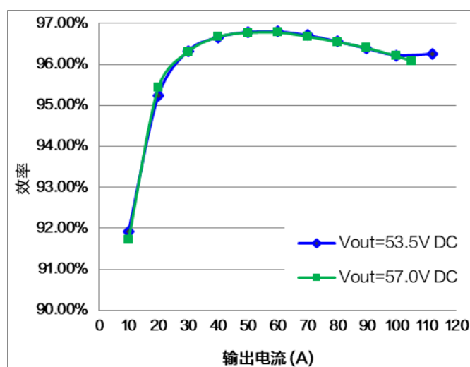
图2 输出效率曲线 (380V AC, 25°C)
