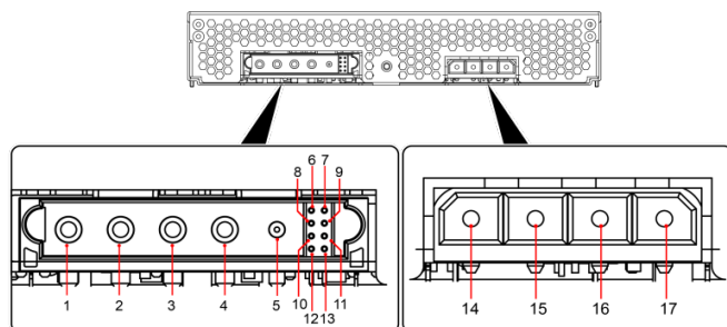
图4 模块端子管脚示意
