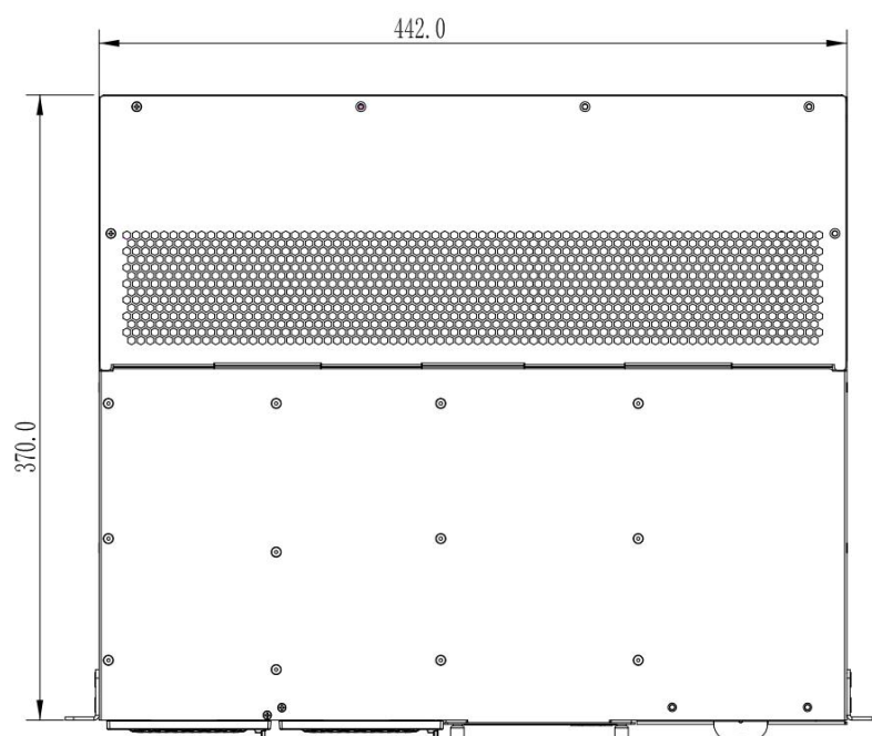
顶视图
