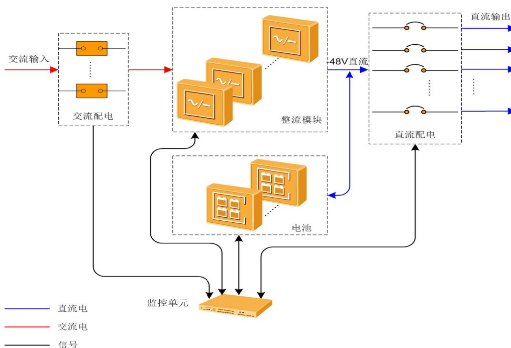
图2-1 电源系统工作原理示意图
