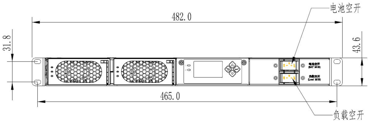
前视图
