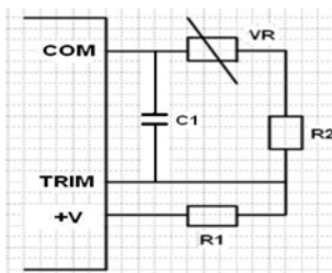
图4 Trim调压接线图
