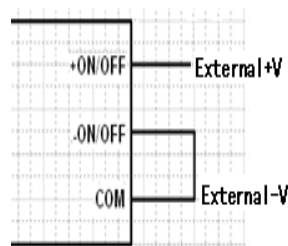
图3 遥控外部供电接线图
