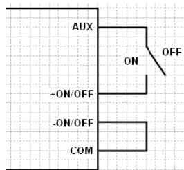
图2 遥控接线图
