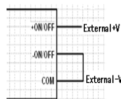
图3 遥控外部供电接线图
