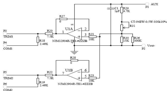
图6 多模块并机均流调压应用连接图
