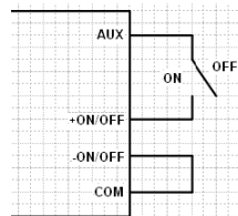
图2 遥控接线图
