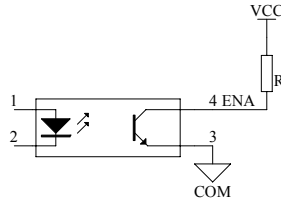
图9 Power On信号应用连接图
