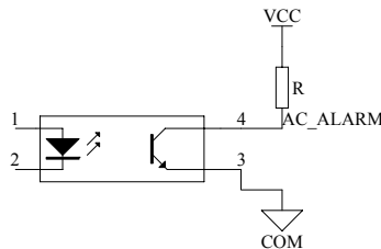
图10 AC_ALARM信号应用连接图
