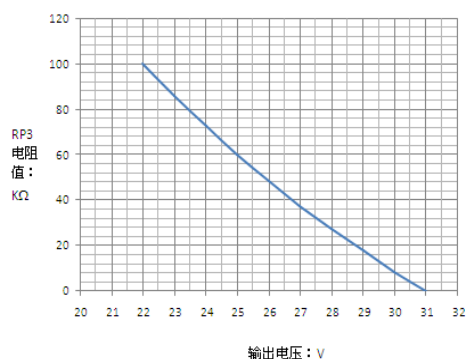
图15 RP3阻值随输出电压的变化关系曲线
