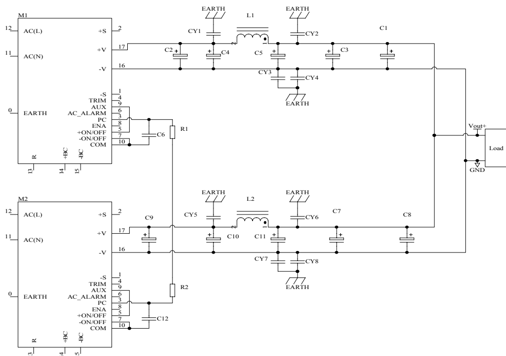
图8 电源并联使用连接方式
