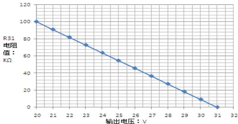
图7 R31阻值随输出电压的变化关系曲线
