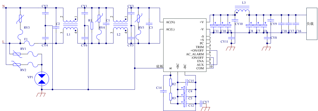
图1 产品应用连线图
