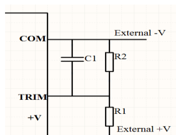
图6 Trim调压接线图
