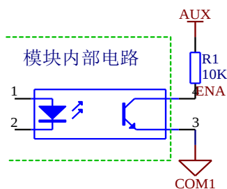
图8 ENA信号连接方式
