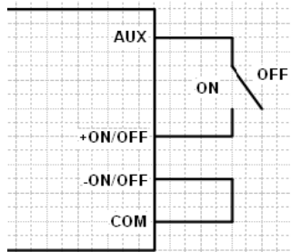
图3 遥控接线图
