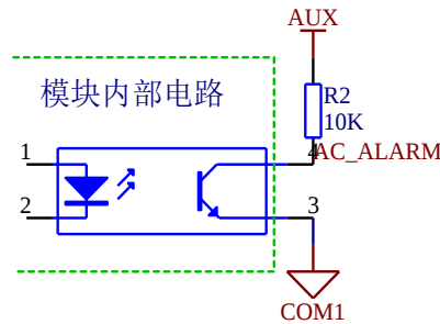
图9 AC_ALARM信号连接方式
