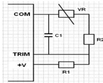
图5 Trim调压接线图
