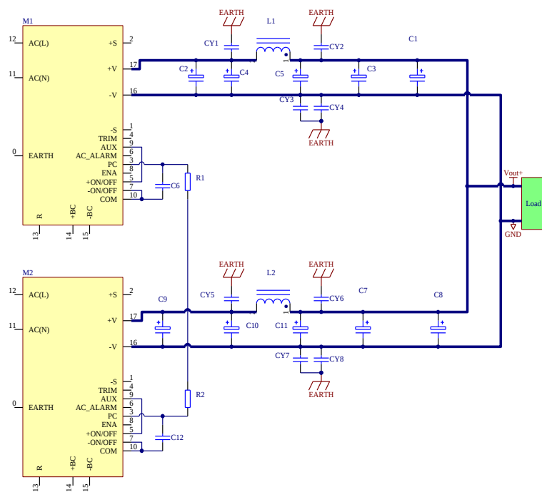
图7 电源并联使用连接方式
