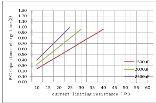
图10 PFC储能电容与防冲击电阻充电时间曲线图
