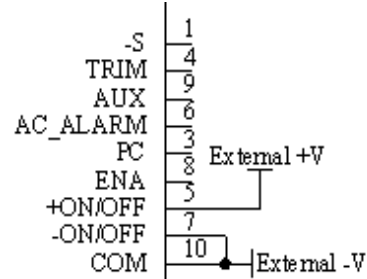
图4 遥控外部供电接线图
