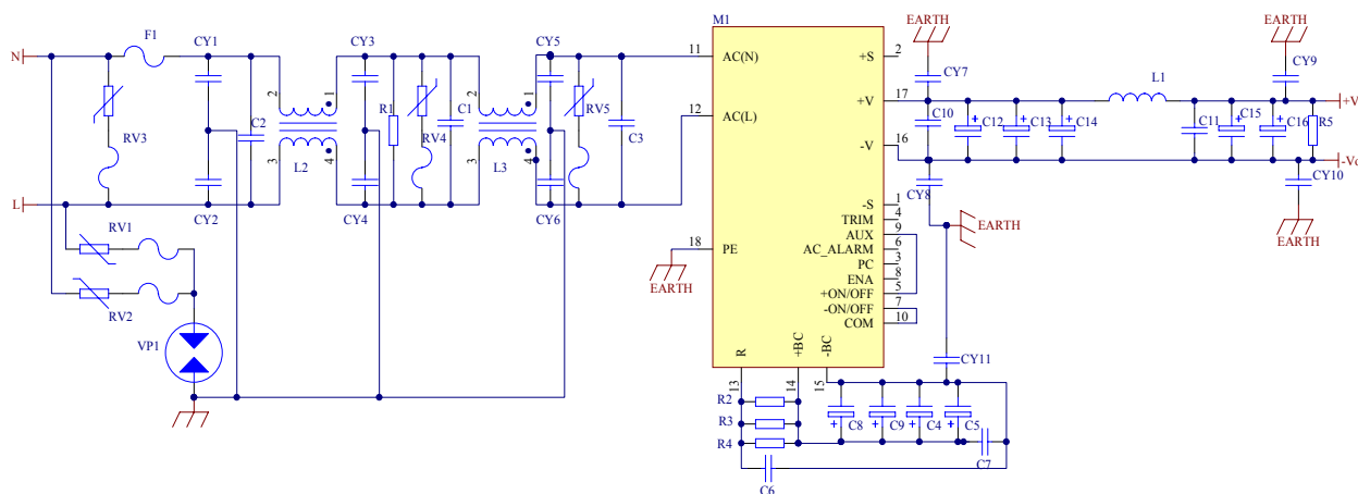
图2 产品应用连线图2
