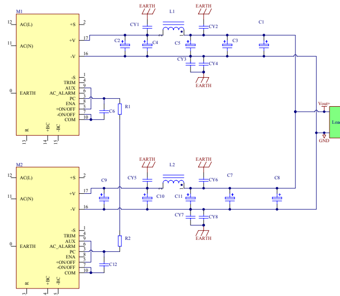
图9 电源并联使用连接方式
