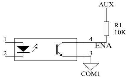
图10 ENA信号连接方式
