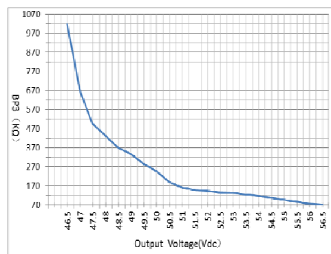
图16 RP3阻值随输出电压的变化关系曲线
