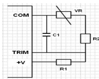
图5 Trim调压接线图
