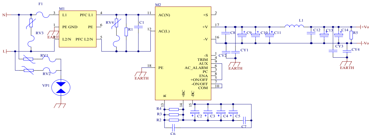
图1 产品应用连线图1
