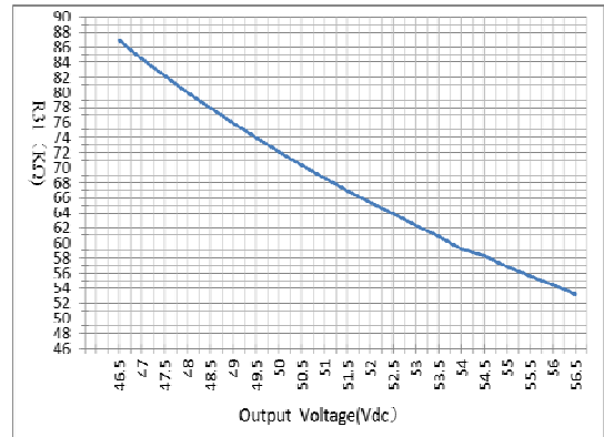
图8 R31阻值随输出电压的变化关系曲线
