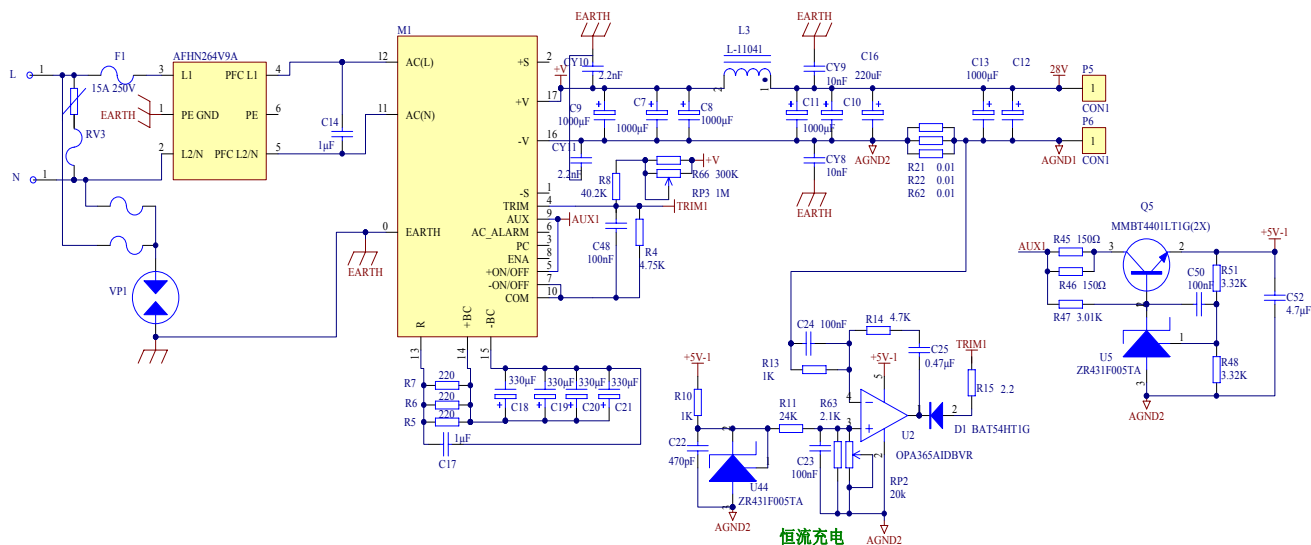
图12 电源恒流充电连接方式
