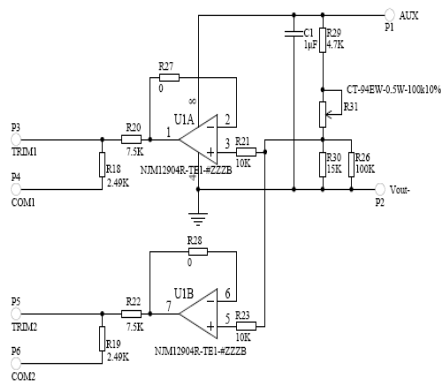
图7 多模块并机均流调压应用连接图
