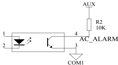
图11 AC_ALARM信号连接方式
