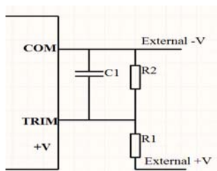
图6 Trim调压接线图
