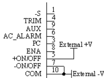
图4 遥控外部供电接线图
