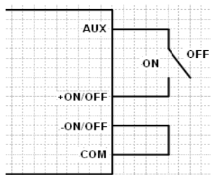
图3 遥控接线图
