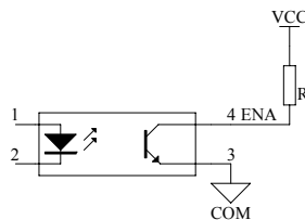
图9 Power On信号应用连接图
