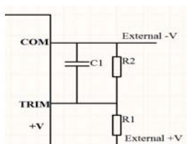
图5 Trim调压接线图
