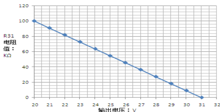
图7 R31阻值随输出电压的变化关系曲线
