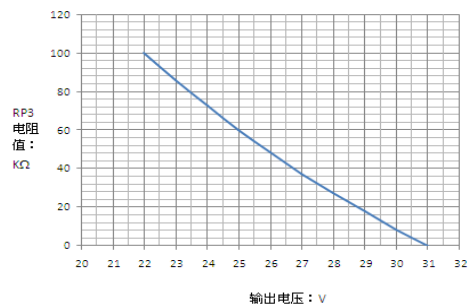
图15 RP3阻值随输出电压的变化关系曲线
