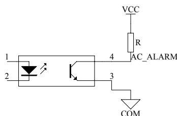
图8 AC_ALARM信号应用连接图
