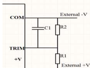
图5 Trim调压接线图
