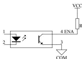
图7 Power On信号应用连接图
