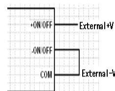
图3 遥控外部供电接线图
