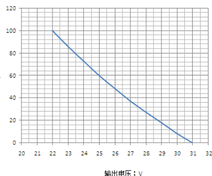
图15 RP3阻值随输出电压的变化关系曲线
