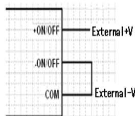
图3 遥控外部供电接线图
