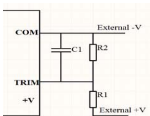
图5 Trim调压接线图
