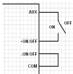
图2 遥控接线图
