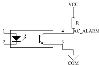
图10 AC_ALARM信号应用连接图
