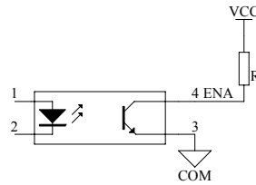
图9 Power On信号应用连接图
