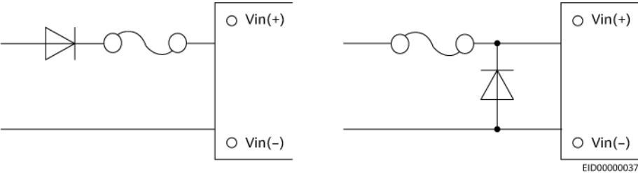
图 3-1 反极性保护电路
