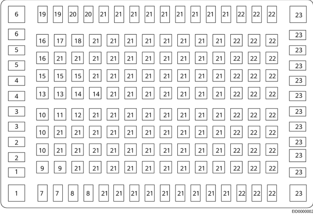
图 5-3 引脚分布（NDD12S55-P1）
