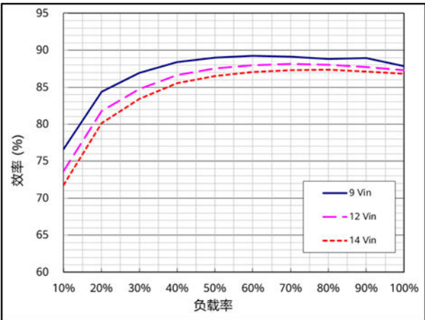
效率 ( T_A=25^{\circ}C , V_{out}=1.0V , I_{out}=400A )
