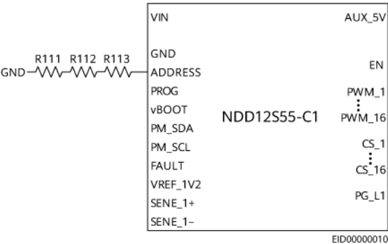
图 8-1 ADDRESS 配置原理图
