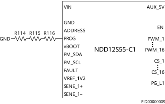
图 5-9 推荐 PROG 配置原理
