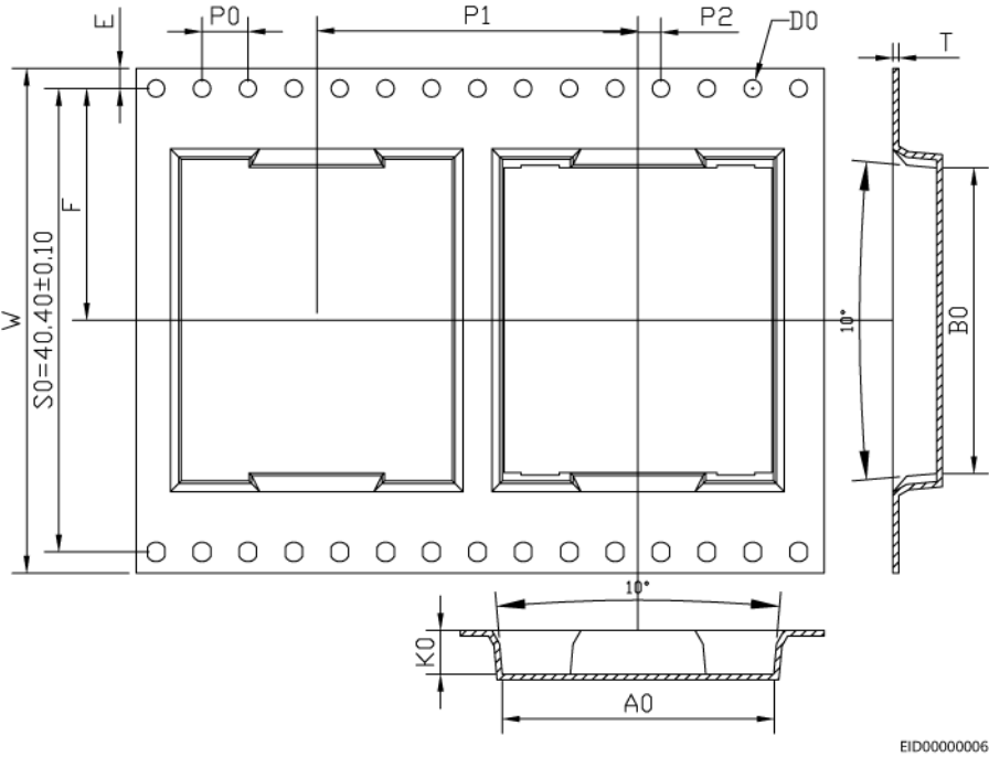
图 11-1 封装信息（NDD12S55-P1）
