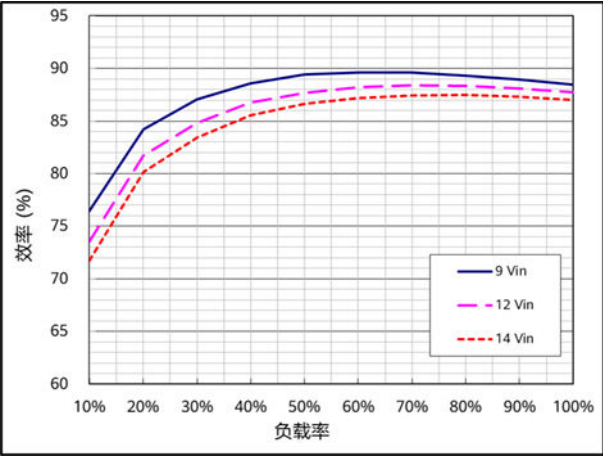
效率 ( T_A=25^{\circ}\text{C} , V_{\text{out}}=1.0\text{V} , I_{\text{out}}=600\text{A} )
