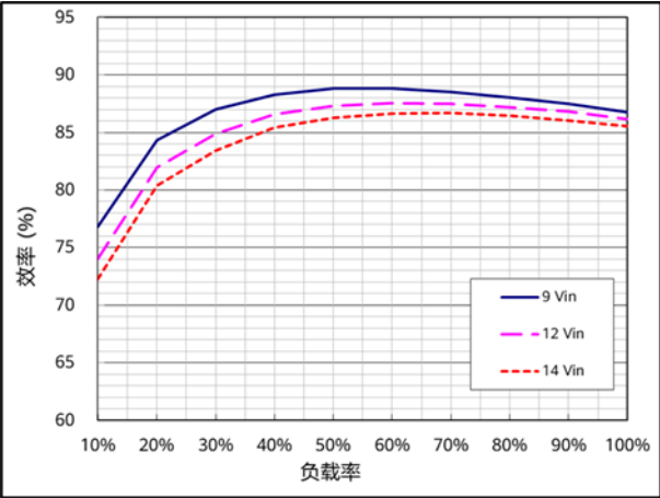
效率 ( T_A=25^{\circ}\text{C} , V_{\text{out}}=1.0\text{V} , I_{\text{out}}=800\text{A} )
