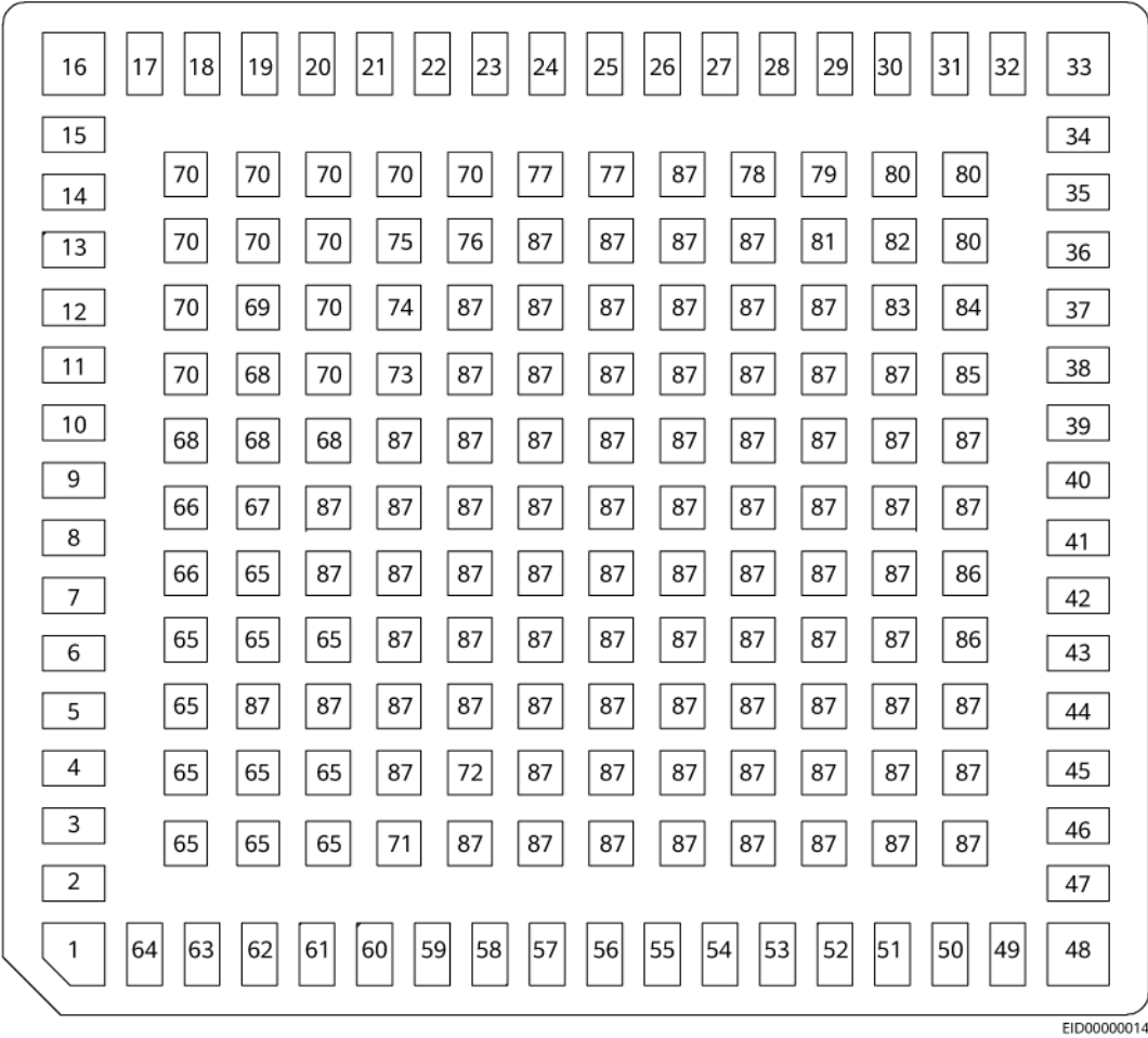
图 5-4 引脚分布（NDD12S55-C1）
