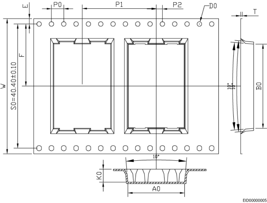
图 11-2 封装信息（ NDD12S55-C1 ）
