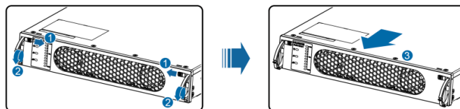
图5 移出模块
