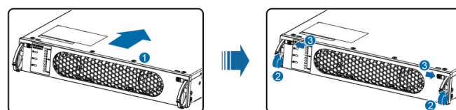
图6 安装模块
