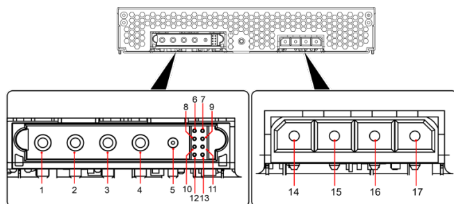
图4 模块端子管脚示意图
