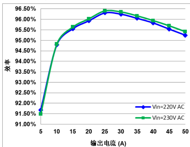
图2 输出效率曲线
