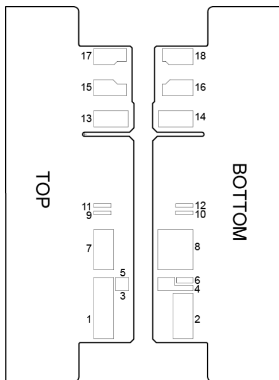
图4 模块金手指示意图
